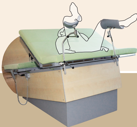
Querbett Mittelteil verstellbar 0–68° Kopftieflage (Trendelenburg) 0–12° Fußtiefelage 0–15°
